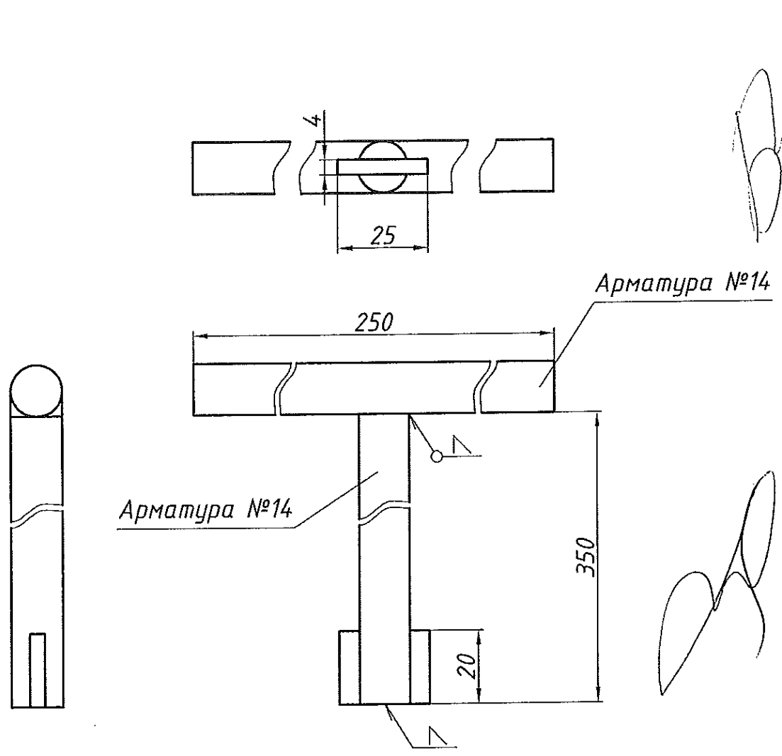
Инструмент за повдигане на капак за електрошахти
