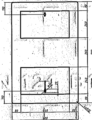
Капак за ЕЛЕКТРОШАХТИ поглед надолу
